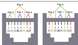
T568A
