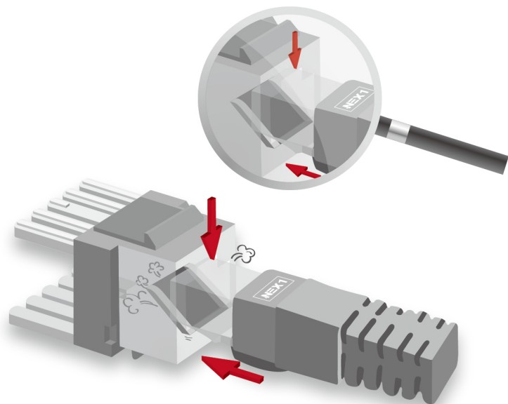
Smart dust cover 智慧防塵蓋/スマート防塵カバー
